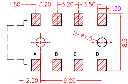
印制板开孔示意图
