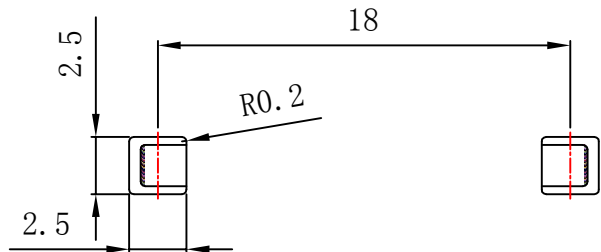
安装尺寸
